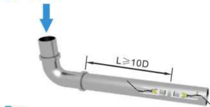
Tee
